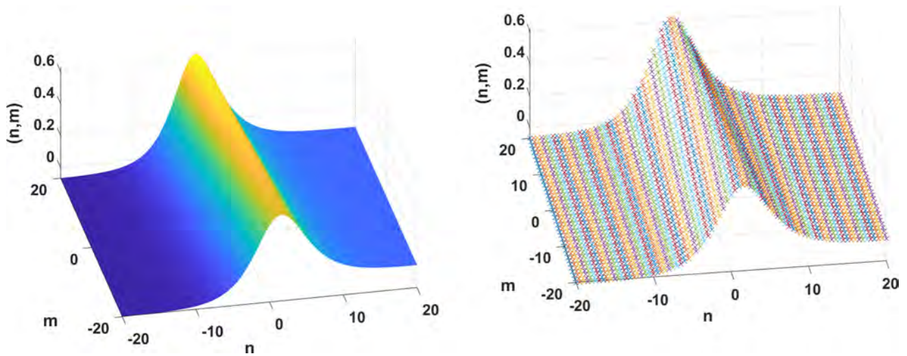
Fig. 3 Bright soliton: for numerical values \eta = 0.7 + 0.54i , q = 3 , b = 2
