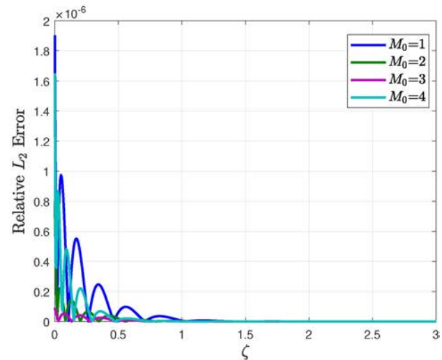
(d) Error
