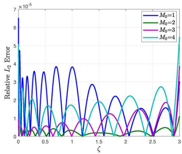
(b) Error
